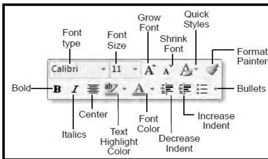
Figure 138: Mini Toolbar
