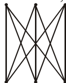
K_{3,3}
