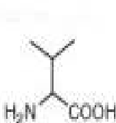
Valine (Val, V)
